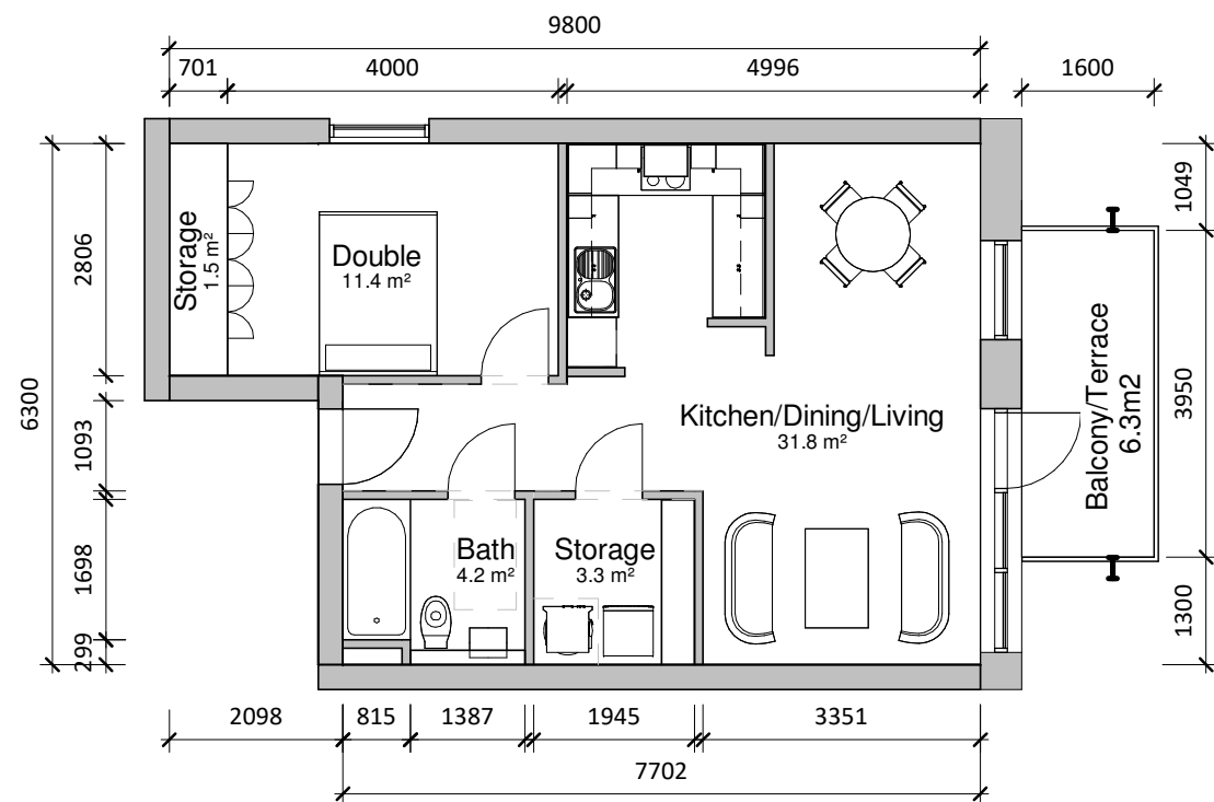
1 1 Bed/2P - 54.4 sqm 1 : 100
