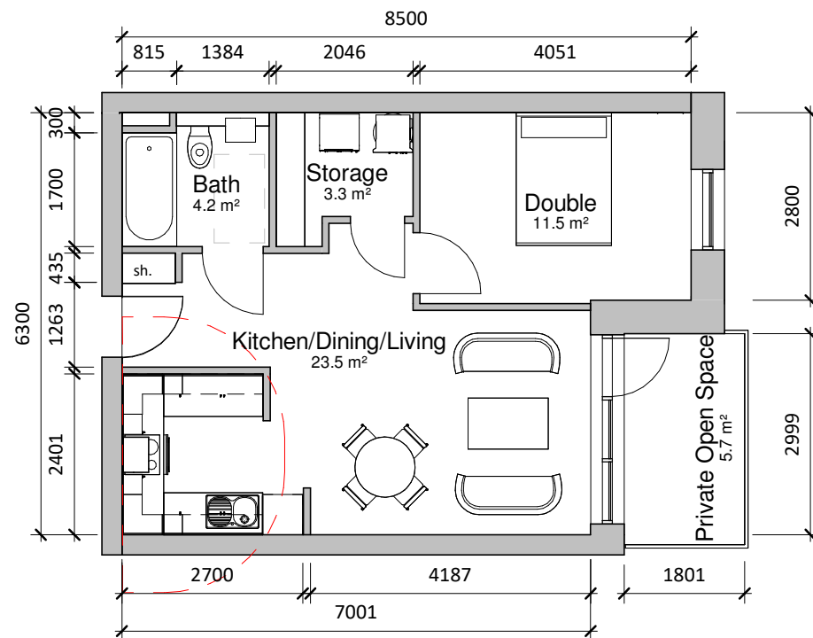
1 1 Bed/2P - 48.4 sqm 1 : 100
